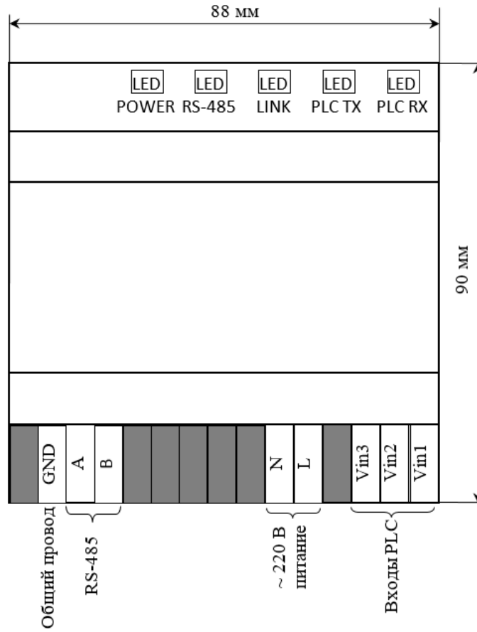
Рисунок 2. Чертеж корпуса базовой станции BS-PLC-501
